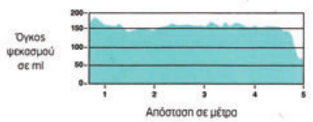
Τυπικό ίχνος ψεκασμού που παράγεται από τα ακροφύσια ΧΤ
